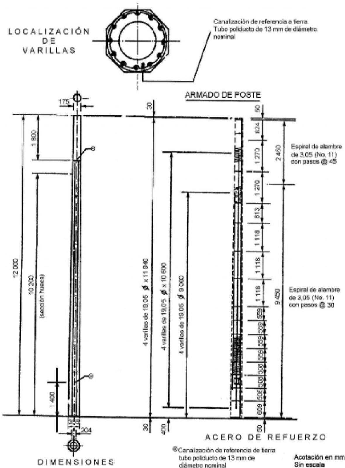
FIGURA 9 – Poste PCR-12-1250
