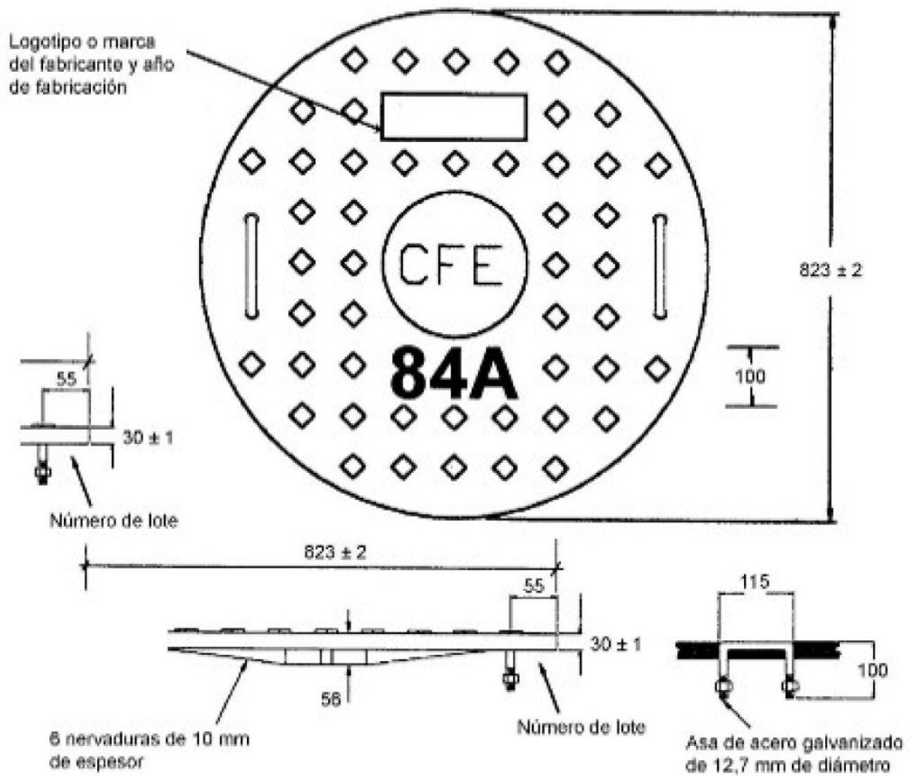
FIGURA 2A - Características y dimensiones de la tapa 84 A
