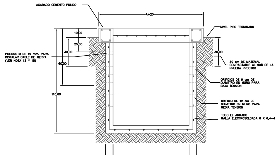
NIVEL FREÁTICO ALTO CORTE B-B'
