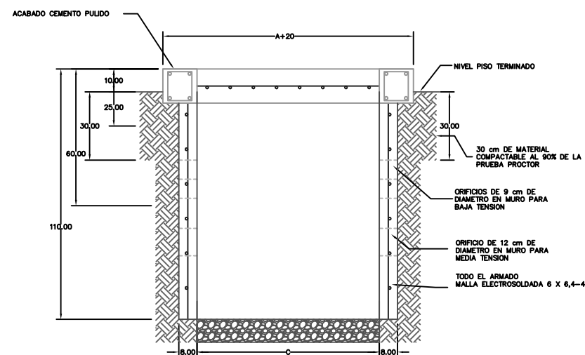
NIVEL FREÁTICO BAJO CORTE B-B'
