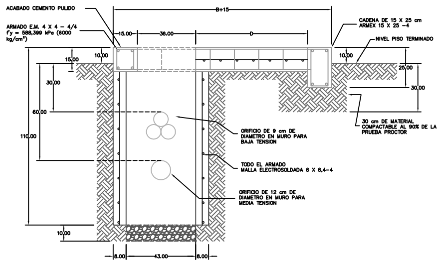
NIVEL FREÁTICO BAJO CORTE A-A'
