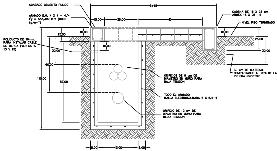
NIVEL FREÁTICO ALTO CORTE A-A'
