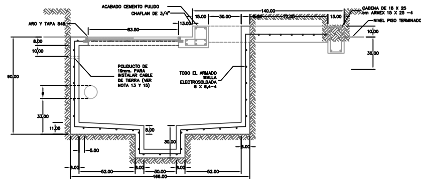
NIVEL FREÁTICO ALTO CORTE A-A'
