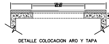
DETALLE COLOCACION ARO Y TAPA
