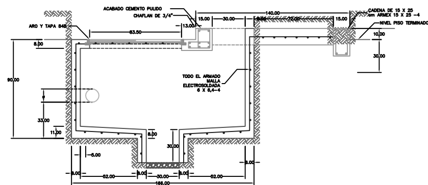
NIVEL FREÁTICO BAJO CORTE A-A'
