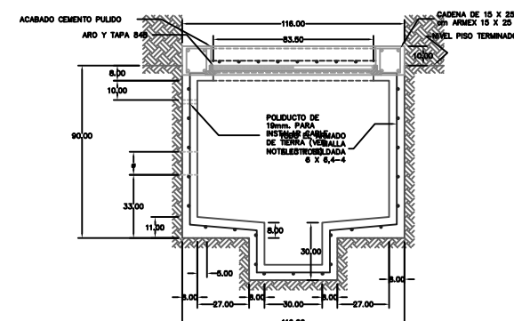
NIVEL FREÁTICO ALTO CORTE B-B'
