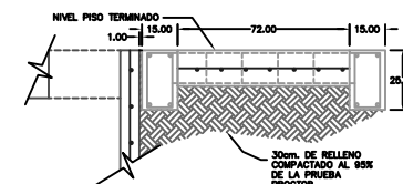
30cm. DE RELLENO COMPACTADO AL 95% DE LA PRUEBA PROCTOR
