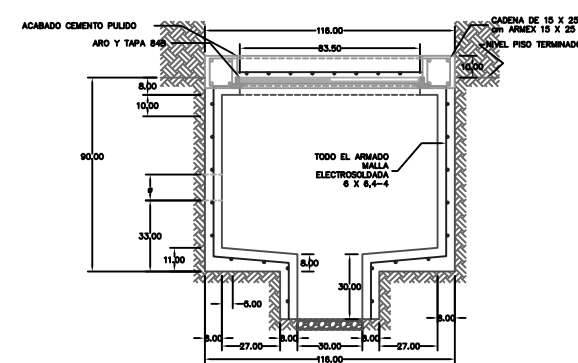
NIVEL FREÁTICO BAJO CORTE B-B'
