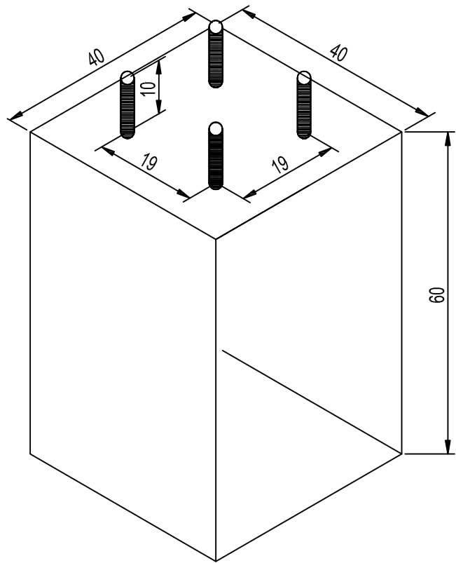
ISOMETRICO
