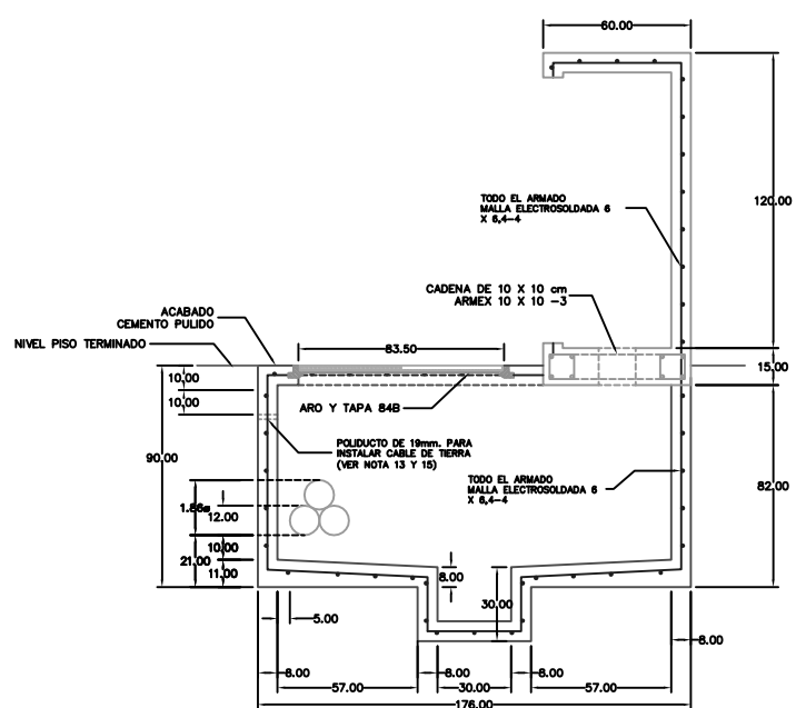
NIVEL FREÁTICO ALTO CORTE A-A'
