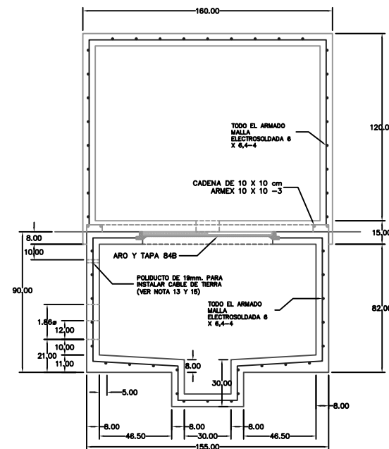
NIVEL FREÁTICO ALTO CORTE B-B'
