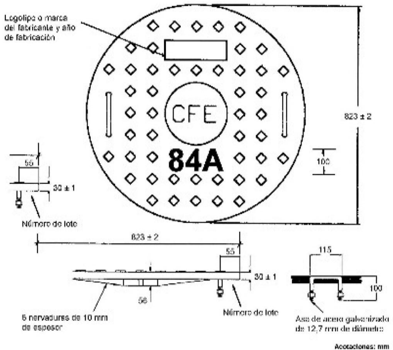
FIGURA 2 – Características y dimensiones de la tapa 84 A
