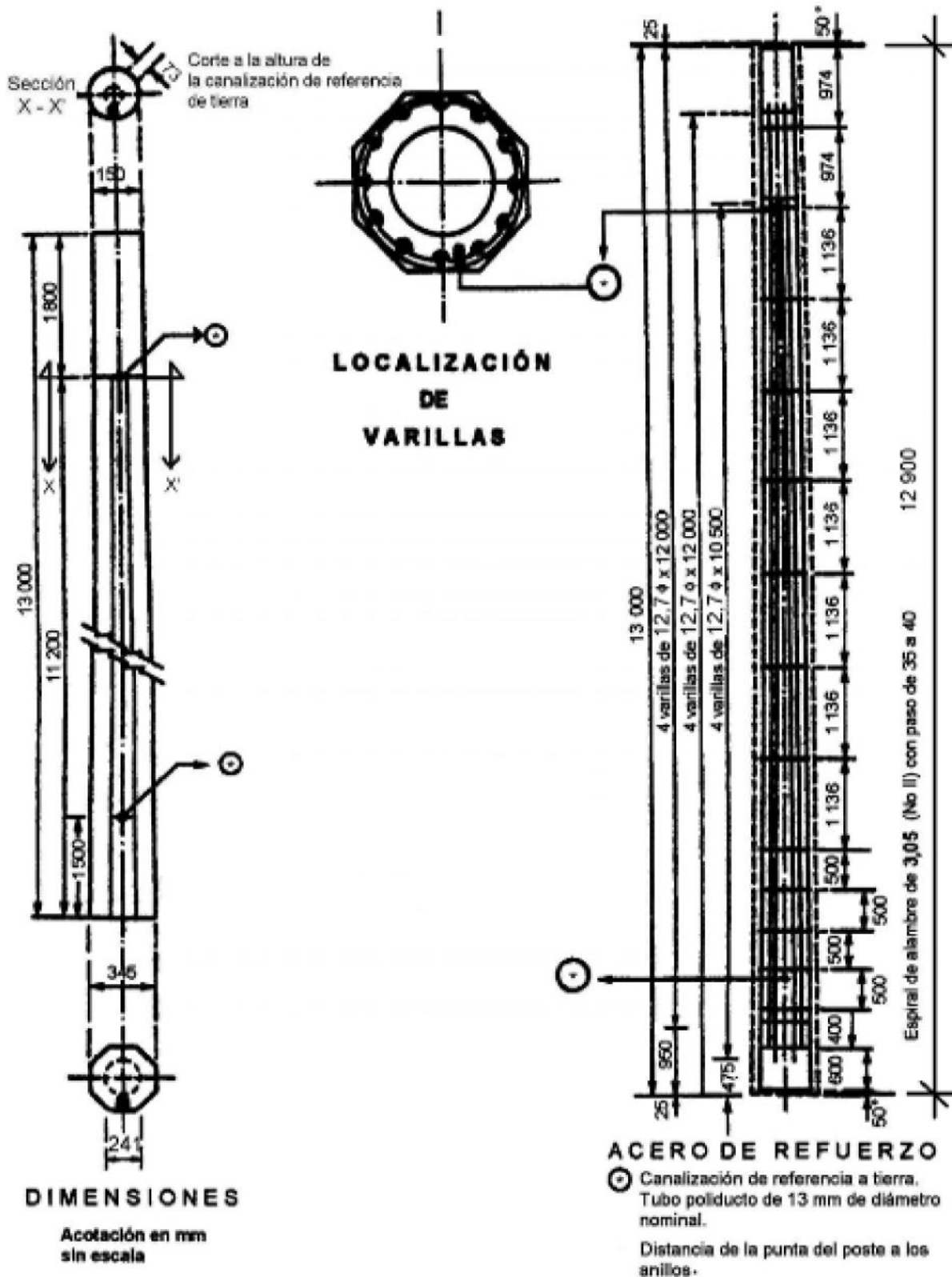
FIGURA 10 – Poste PCR-13-600
