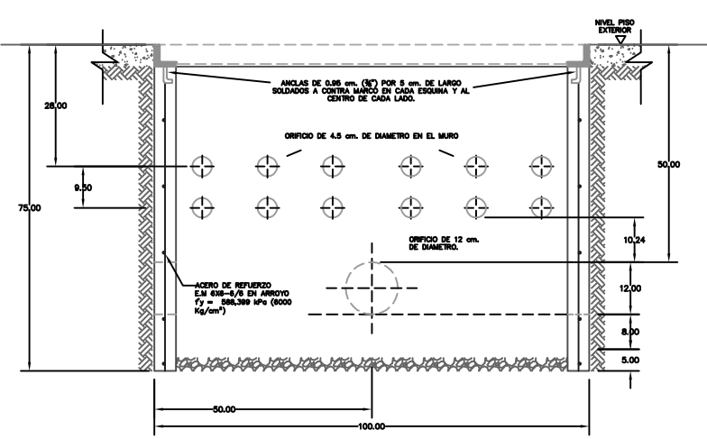
REGISTRO SIN FONDO PARA NIVEL FREATICO BAJO
