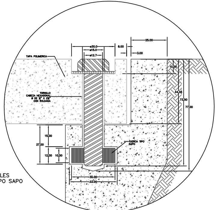
REGISTRO SIN FONDO PARA NIVEL FREATICO BAJO
