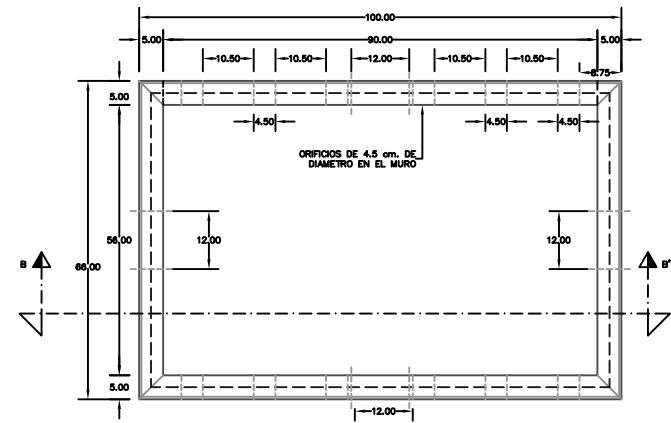
PLANTA REGISTRO SIN FONDO
