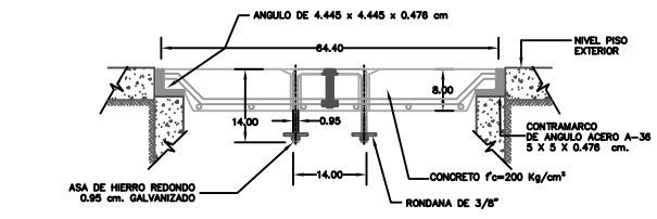
DETALLE TAPA: CORTE D-D'
