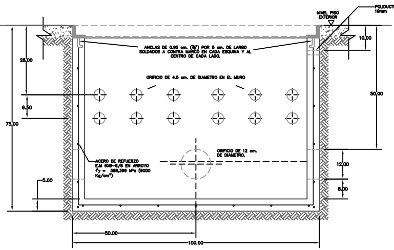
REGISTRO CON FONDO PARA NIVEL FREATICO ALTO
