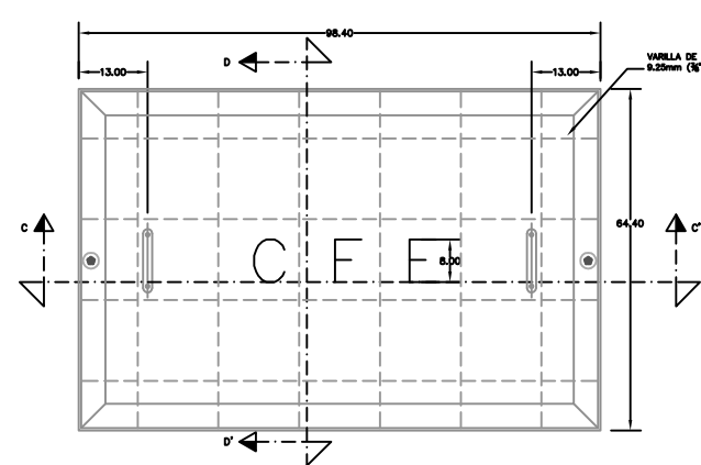
PLANTA TAPA
