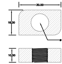
DETALLE TAPA POLIMERICA
