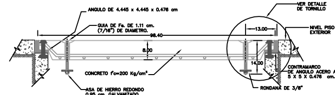
DETALLE TAPA: CORTE C-C'
